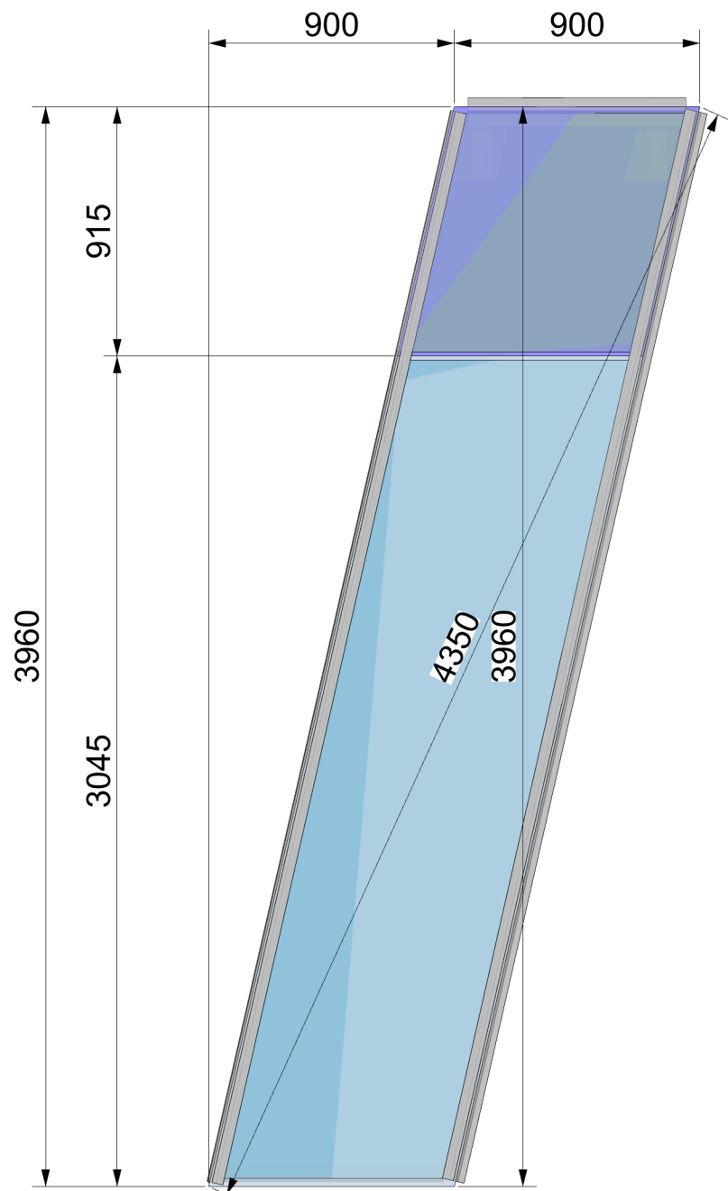
ELEVATION
